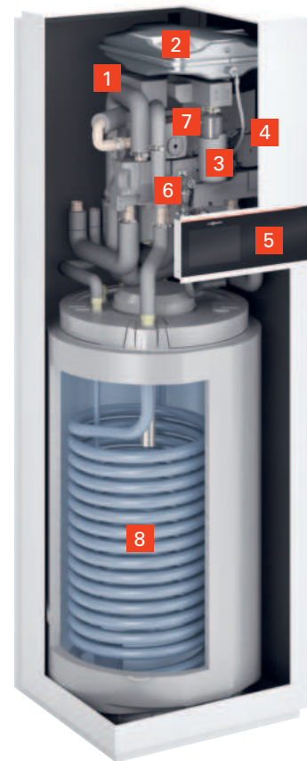
VITOCAL 151-A Inneneinheit
